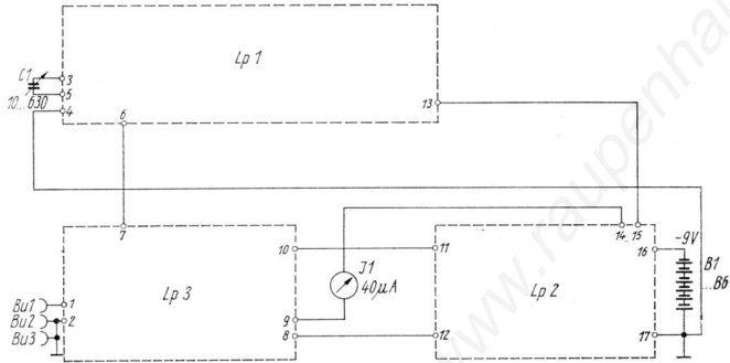
Kapazitätsmeßgerät 1512a - Übersicht
