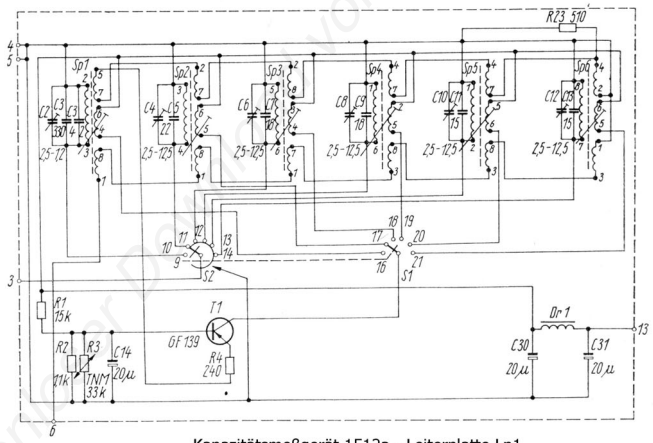
Kapazitätsmeßgerät 1512a - Leiterplatte Lp1
